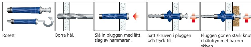
Expansionsankare med krok
