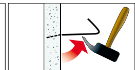
Kroken demonteras enkelt. Vipp upp kroken och tryck den rätt ut.
